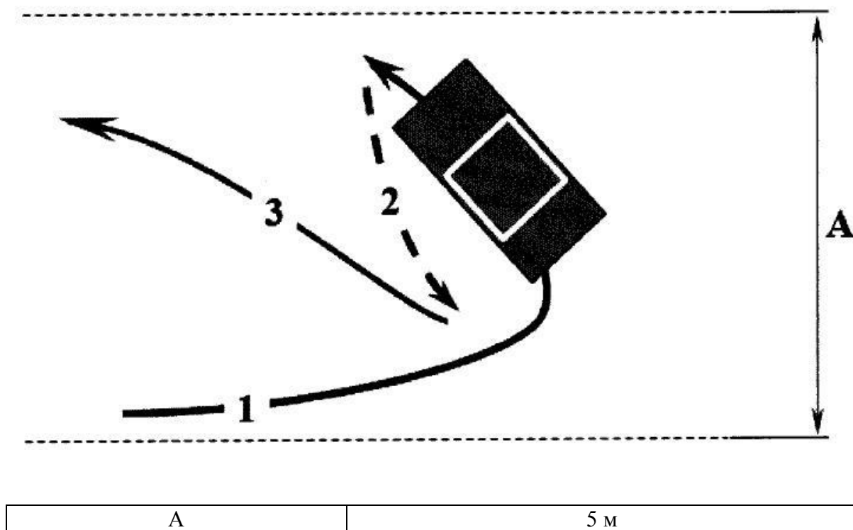
Рисунок 7. Схема маневра "Разворот транспортного средства в ограниченном пространстве (при ограниченной ширине проезжей части) с использованием движения задним ходом"
