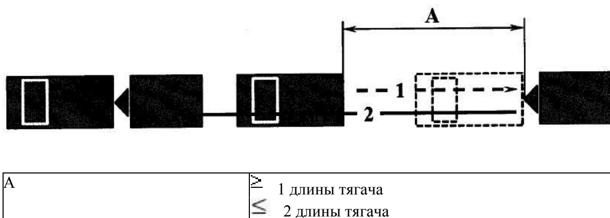
Рисунок 9. Схема и размеры маневра "Сцепление и расцепление или расцепление и повторное сцепление прицепа с тягачом (для транспортных средств категорий "BE", "CE" и "DE" и подкатегорий "C1E" и "D1E", за исключением сочлененных автобусов)" при сцеплении прицепа с тягачом
