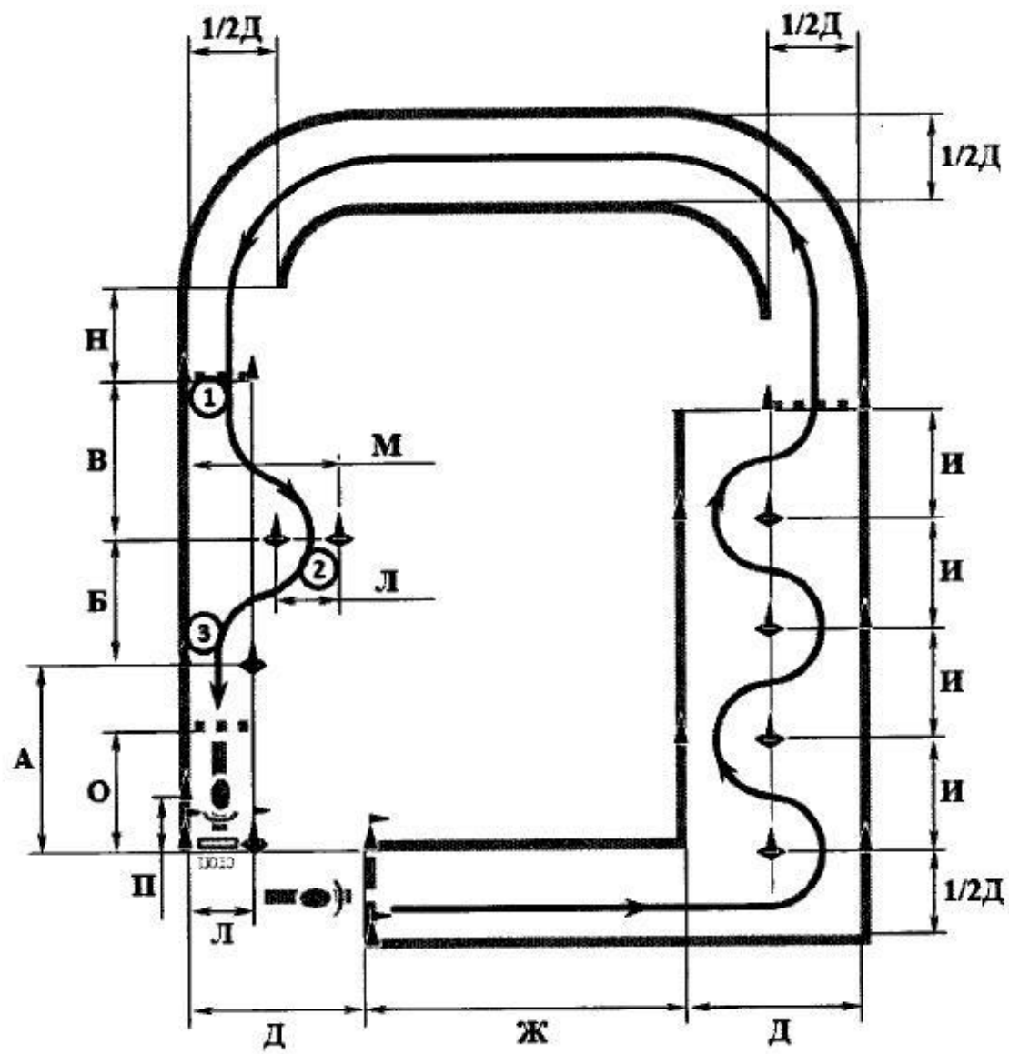
Рисунок 5. Схема "Б" упражнения N 4.
